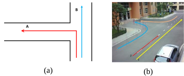
Hình 2. Sự không phù hợp khi sử dụng khoảng cách Hausdorff đo độ tương tự giữa các quỹ đạo
