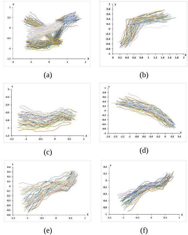
Hình 7. Phân nhóm các quỹ đạo. (a): Tập 250 quỹ đạo; (b): Nhóm 1; (c): Nhóm 2; (d): Nhóm 3; (e): Nhóm 4; (f): Nhóm 5
