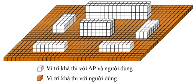
Hình 3. Mô hình hóa vùng không gian lắp đặt mạng WMN thành các khối chức năng.
