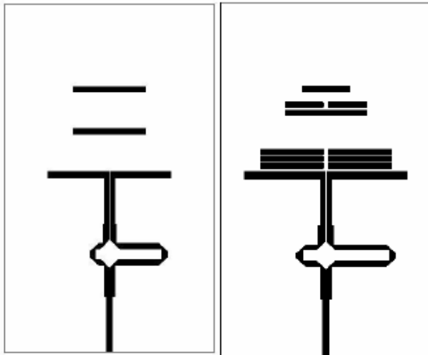
(c) Couple of directors (d) Complex directors
