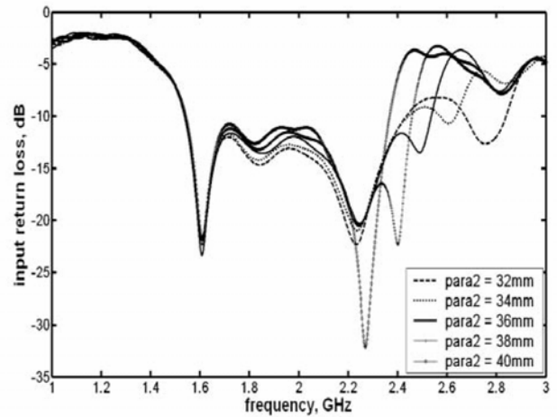
Fig.9. Simulation results of various values of parameter 2- L_{dir}
